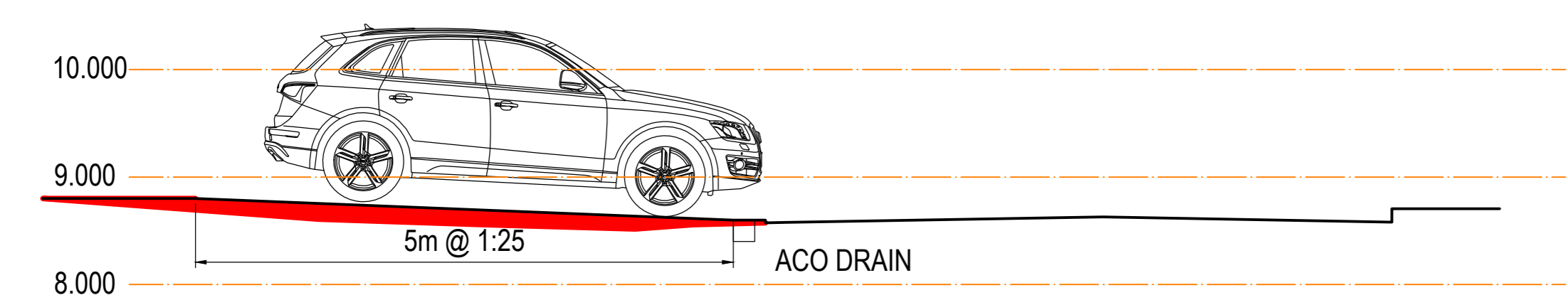
SECTION 'A'
